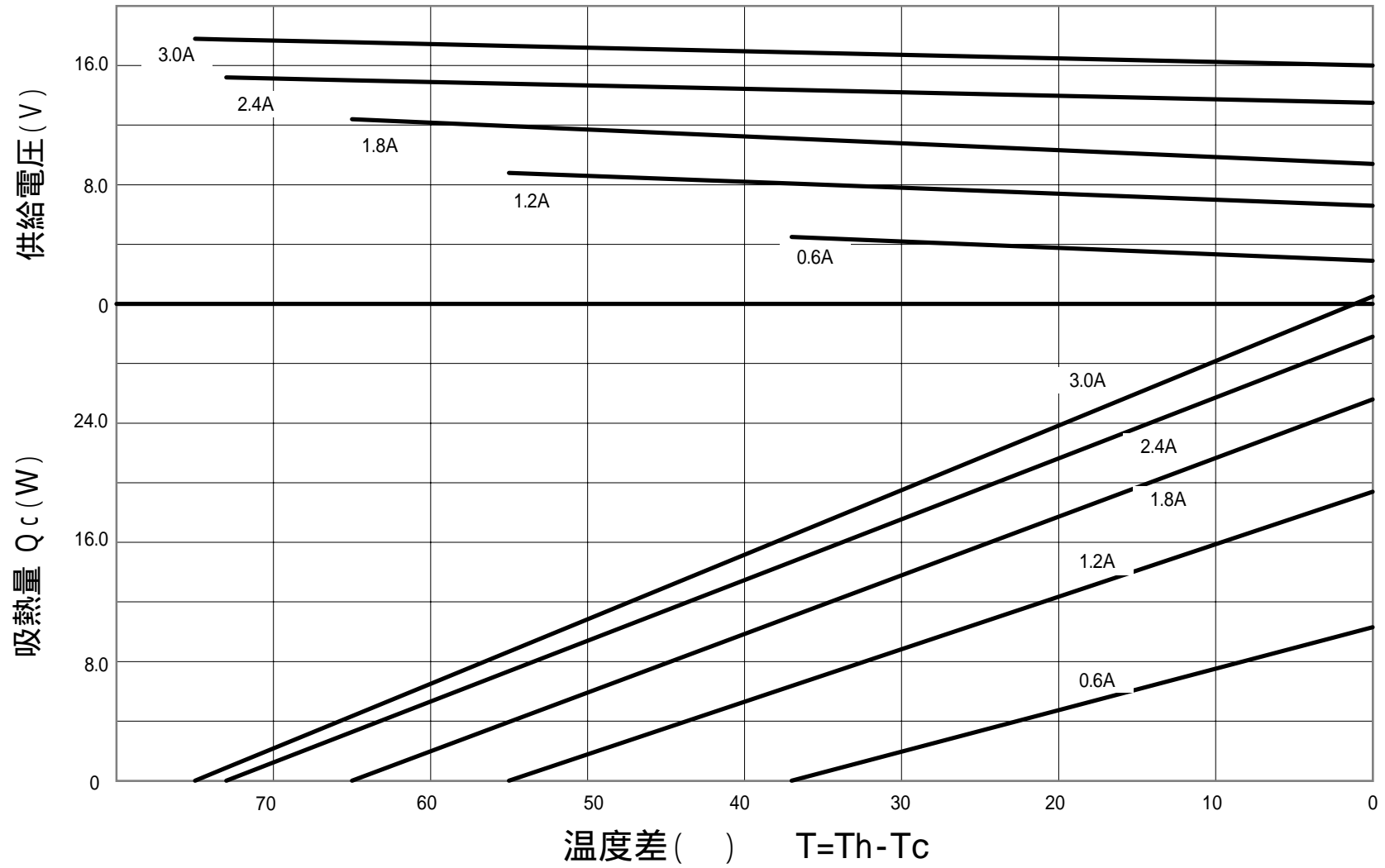
FPH1 - 12703M 特性図 (Th=50 )
