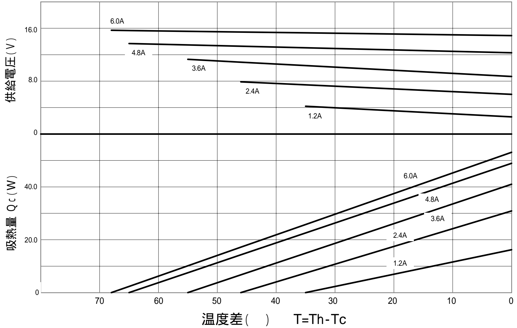
FPH1 - 12706M 特性図(Th=27 )
