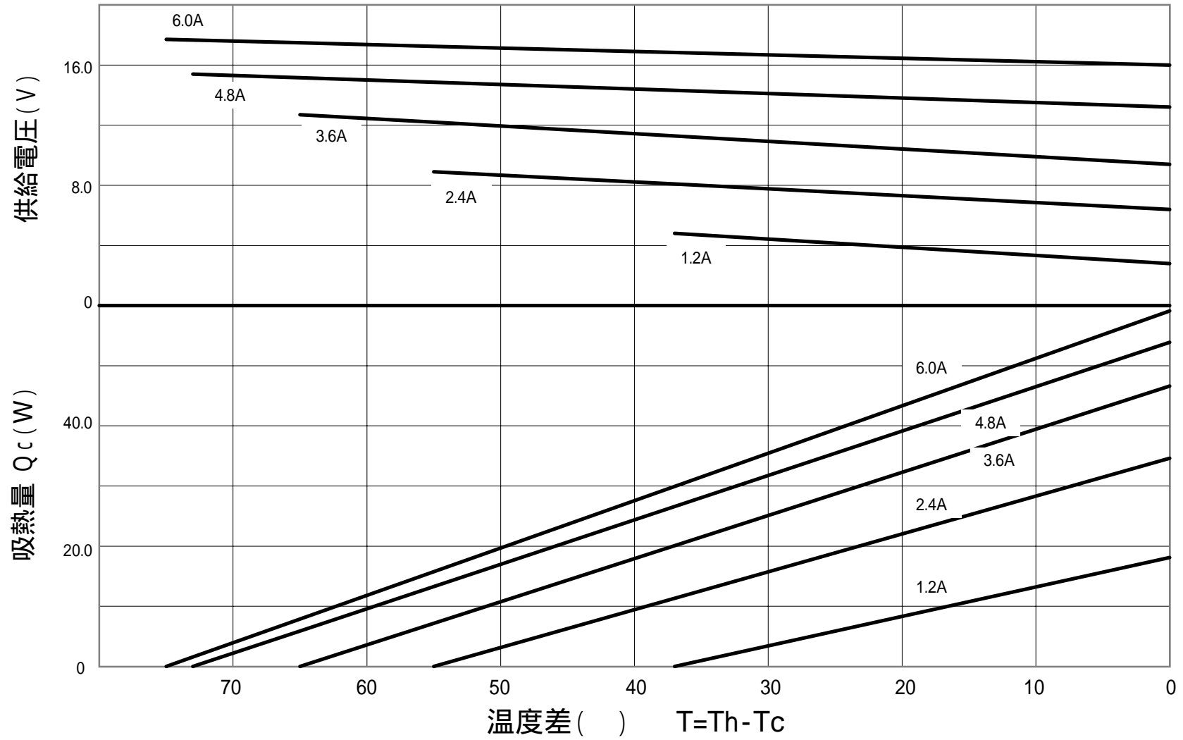
FPH1 - 12706M 特性図 (Th=50 )
