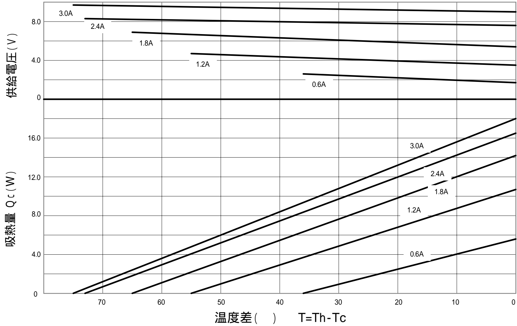
FPH1 - 7103M 特性図 (Th=50 )
