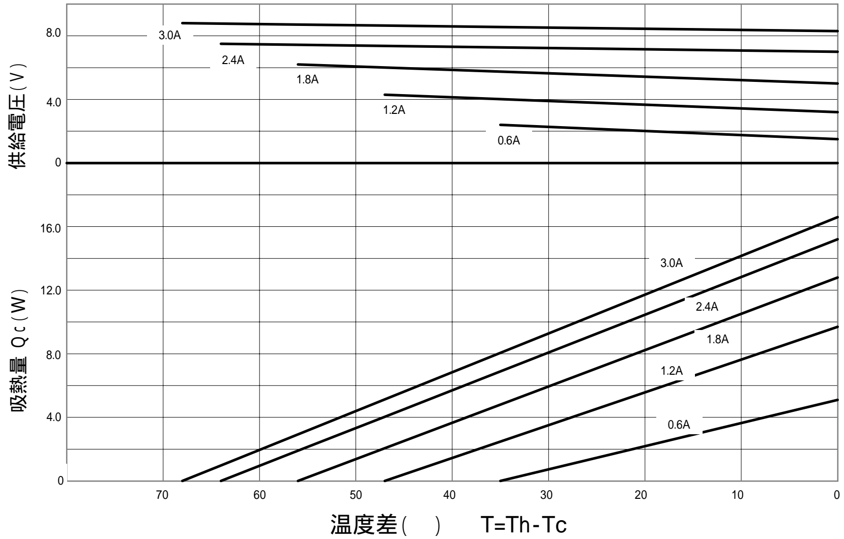
FPH1 - 7103M 特性図(Th=27 )
